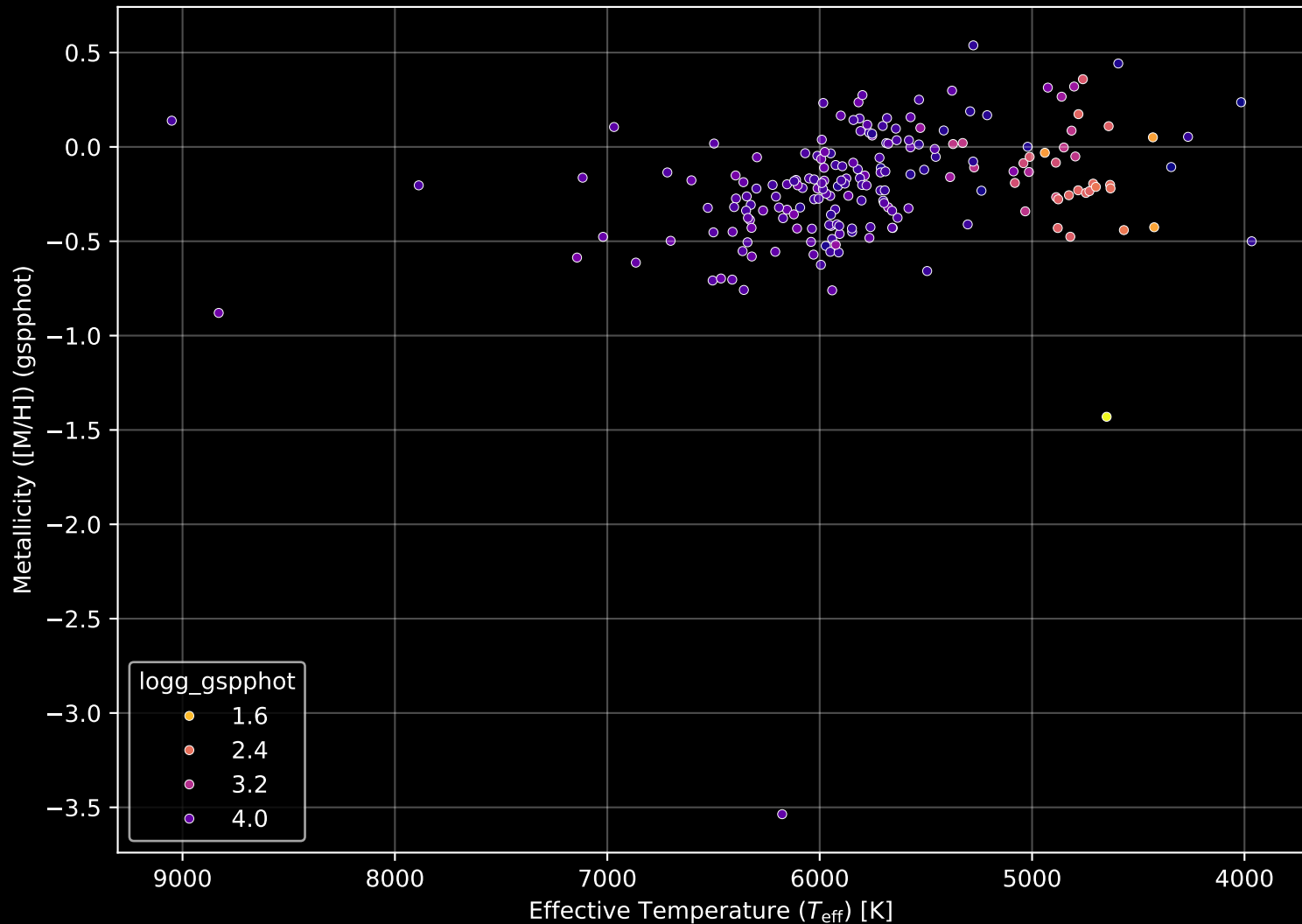
GALAH DR4 Field: [7157] Stellar Population Parameters (n= 195)
