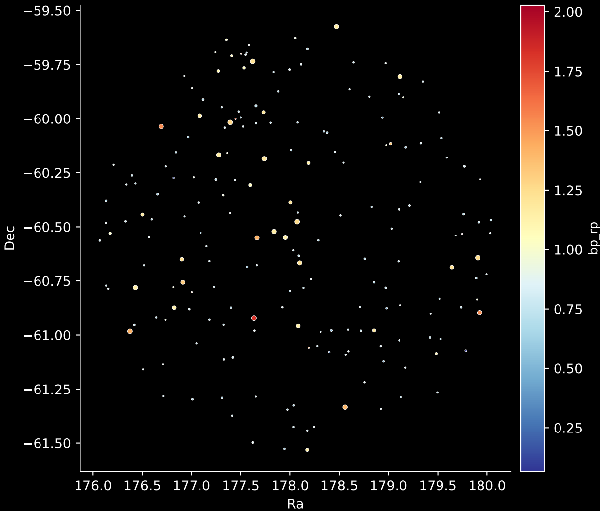
GALAH DR4 Field: [7157] Stars: 195
