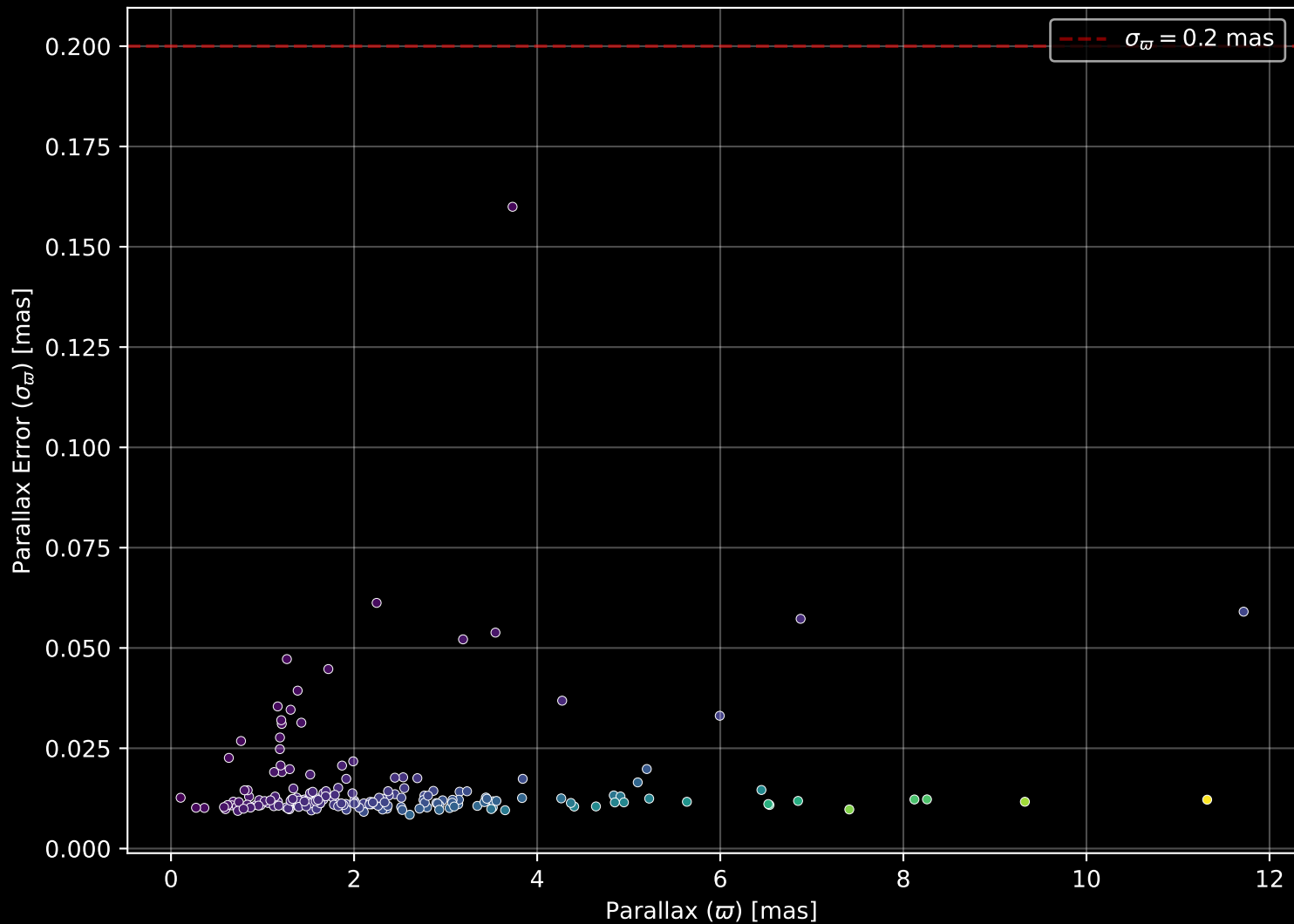
GALAH DR4 Field: [7157] Parallax Quality (n= 195)
