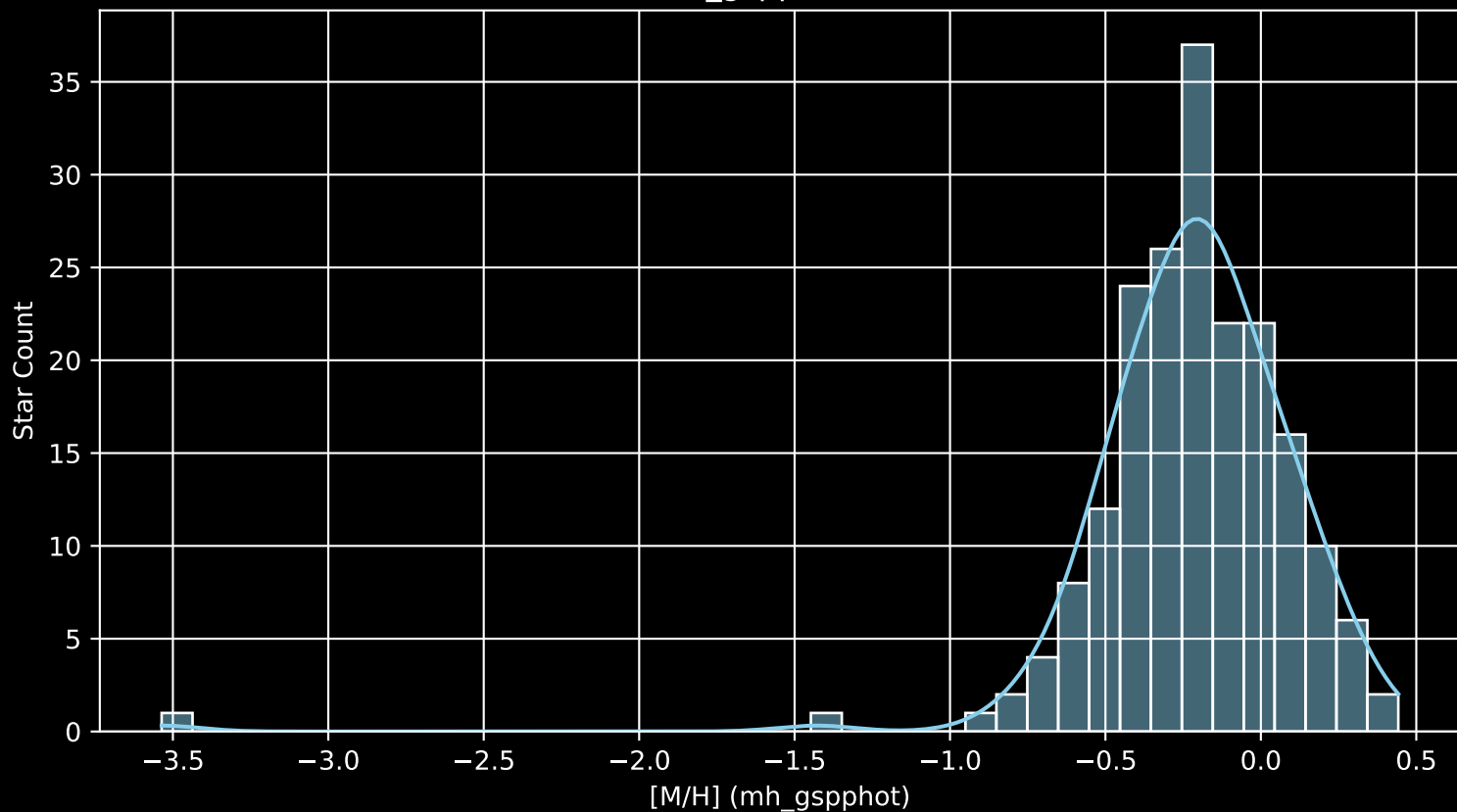
GALAH DR4 Field: [7157] [M/H] (mh_gspphot) (n= 194)
